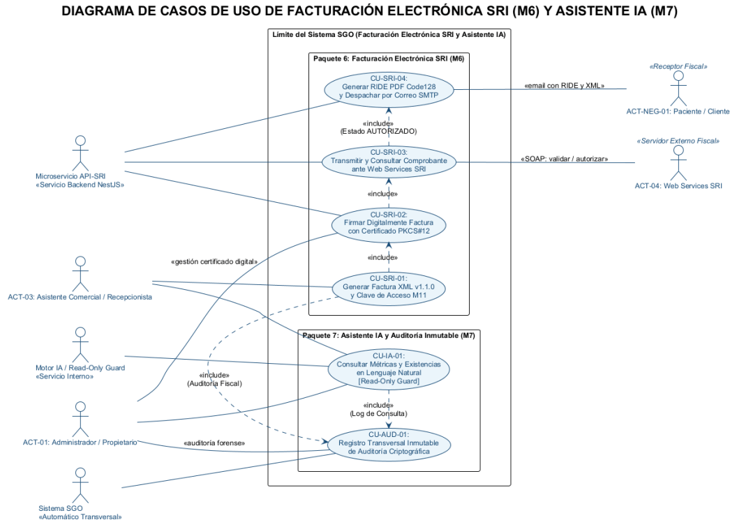
Figura 3.6: Diagrama de Casos de Uso de Facturación Electrónica SRI (M6) y Asistente IA (M7).
