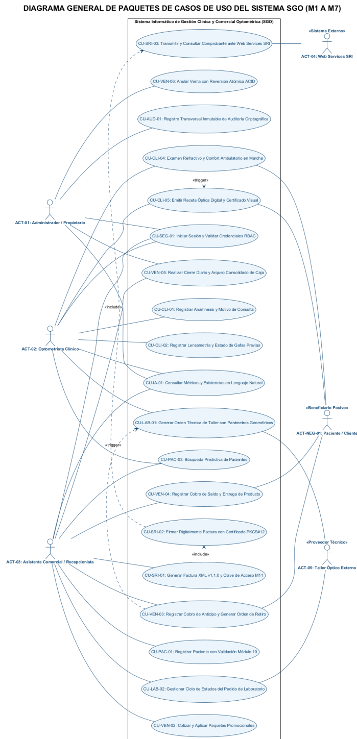
Figura 3.1: Diagrama General de Paquetes de Casos de Uso del Sistema SGO (M1 a M7).
