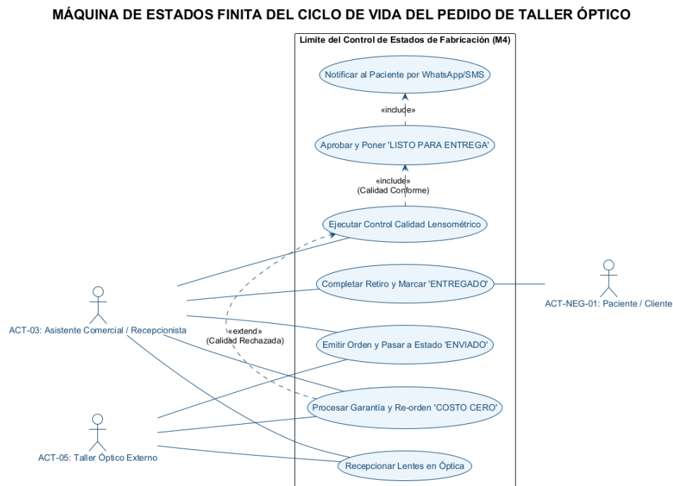
Figura 3.5: Máquina de Estados Finita del Ciclo de Vida del Pedido de Taller Óptico.
