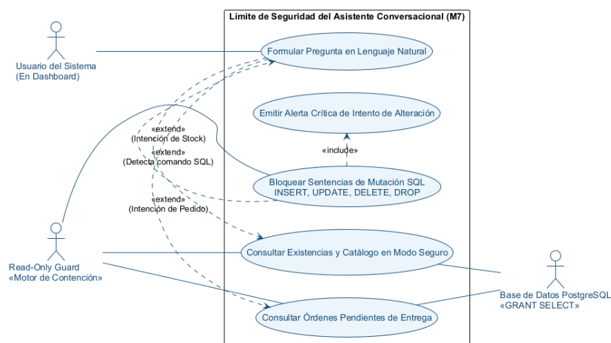
Figura 3.7: Arquitectura de Blindaje de Seguridad Read-Only Guard para el Asistente IA.
