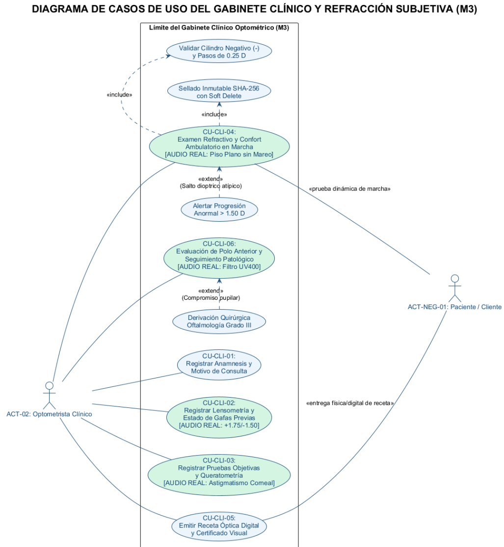
Figura 3.3: Diagrama de Casos de Uso del Gabinete Clínico y Refracción Subjetiva (M3).
