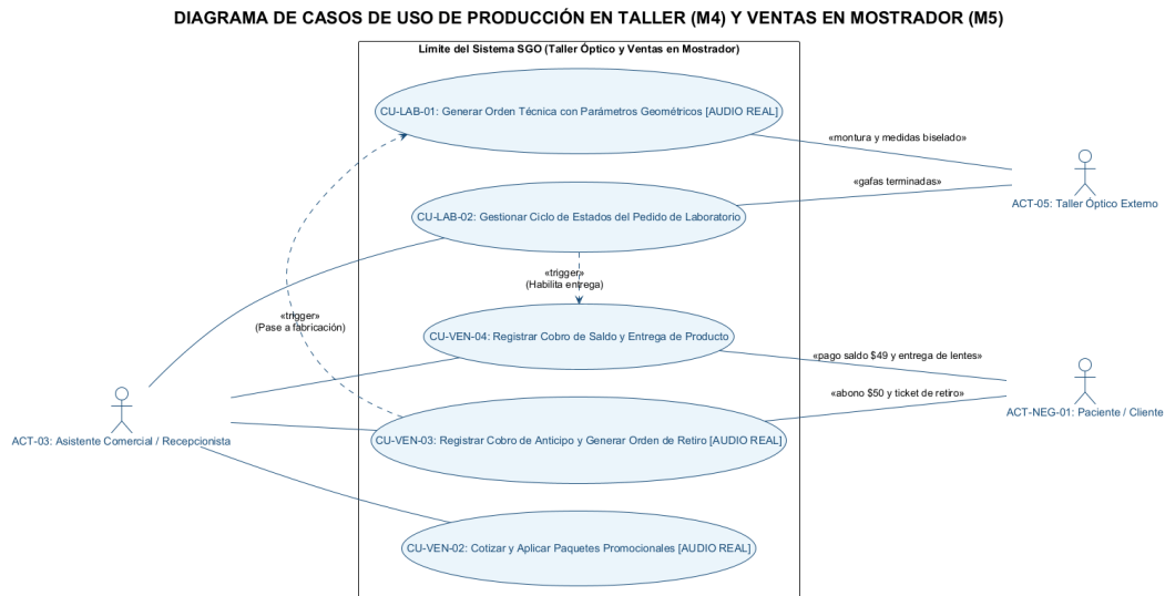
Figura 3.4: Diagrama de Casos de Uso de Producción en Taller (M4) y Ventas en Mostrador (M5).
