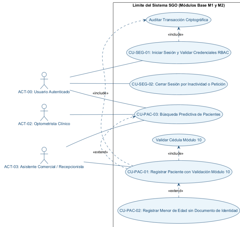
DIAGRAMA DE CASOS DE USO DE ACCESO, SEGURIDAD (M1) Y DEMOGRAFÍA DE PACIENTES (M2)
